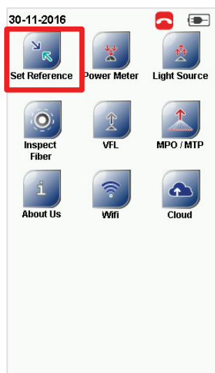
[TOOLS]
