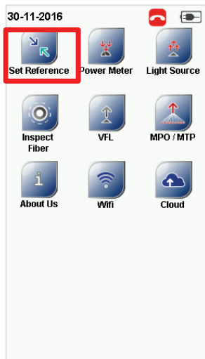
[TOOLS]
