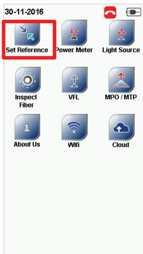
[TOOLS]
