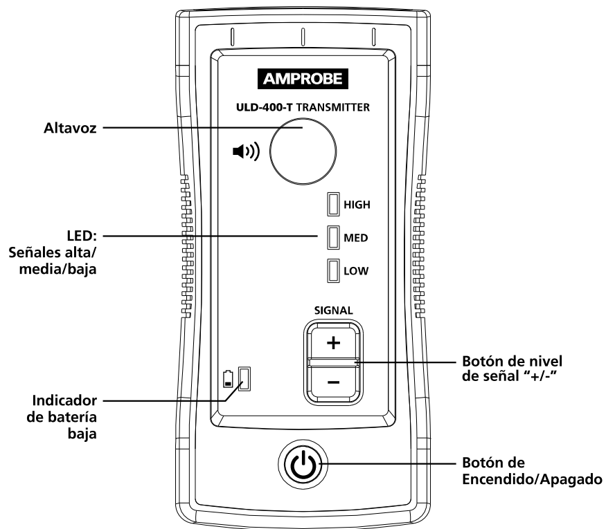
Figura 3.3: Transmisor ULD-400-T
