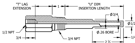
Lagging
