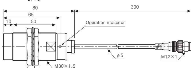
●PRWL30-15A□
