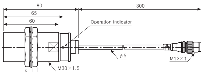
●PRWL30-10A□
