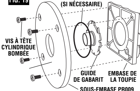
FIG. 20 JOINT TORIQUE EN CAOUTCHOUC (SI NÉCESSAIRE)
