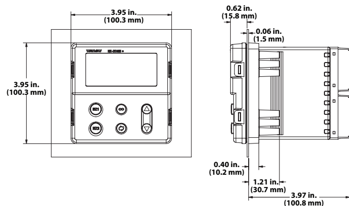
EZ-ZONE PM \frac{1}{4} DIN
