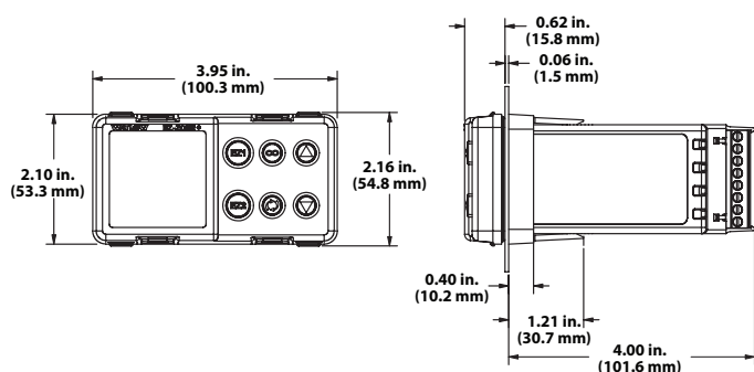
EZ-ZONE PM \frac{1}{8} DIN - Horizontal
