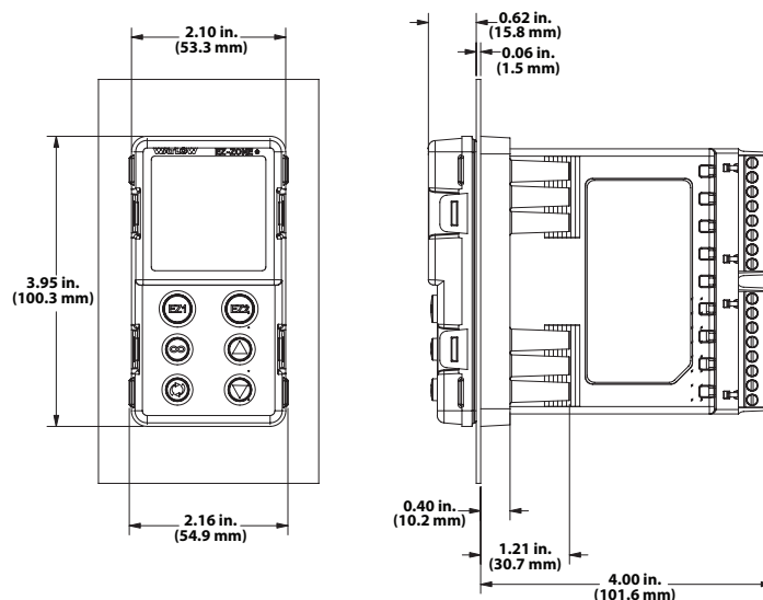
EZ-ZONE PM \frac{1}{8} DIN - Vertical
