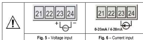
Fig. 5 – Voltage input
