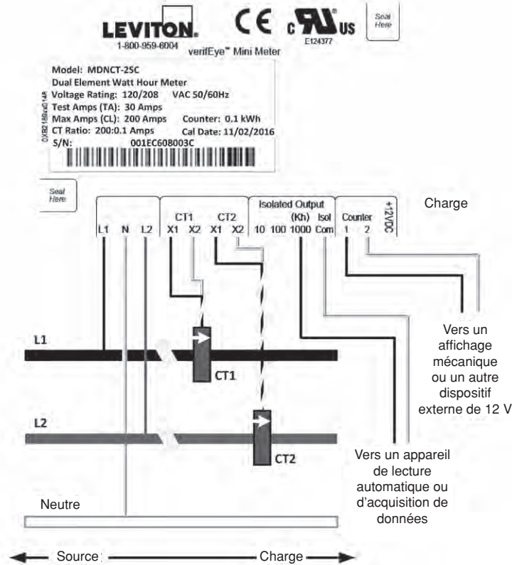
Figure 3 – Raccords d'un minicompteur
