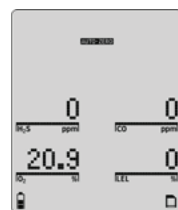
GasAlertMicro 5 IR
