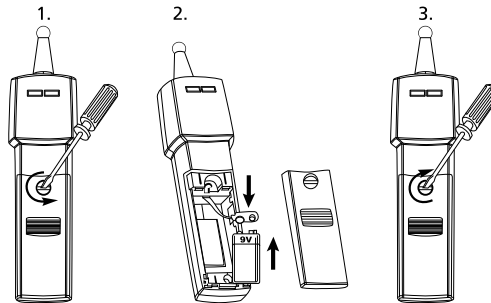
Figur 12: Byta batteri
