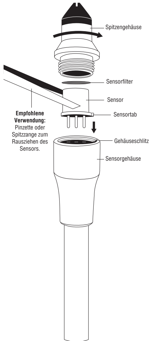
Abbildung: Sensoraustausch
