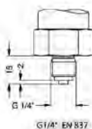
G1/4" EN 837
