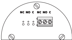
SPDT
