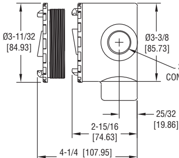
CSA, ATEX Conduit Enclosure
