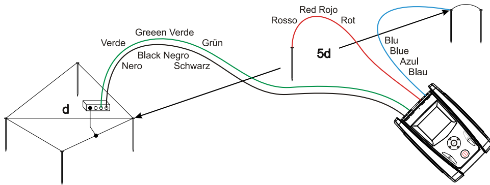
Fig. 6: Medición de la resistencia de tierra - anillos de pequeñas dimensiones
