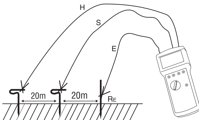
Figura 4: misurazione tripolare
