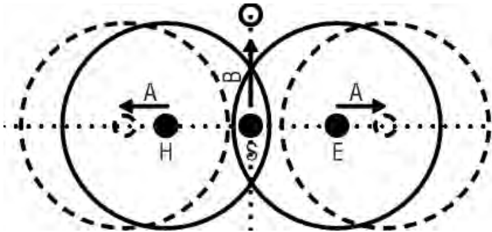
Bild 5: Spannungstrichter
