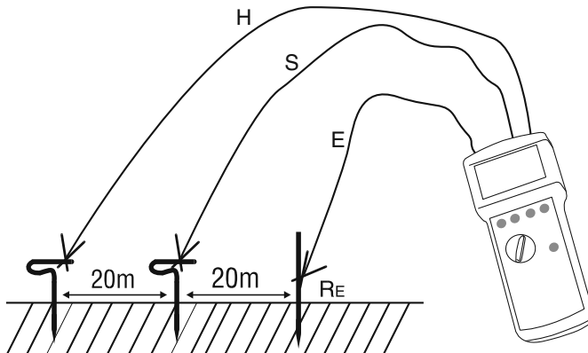
Bild 4: dreipolige Messung
