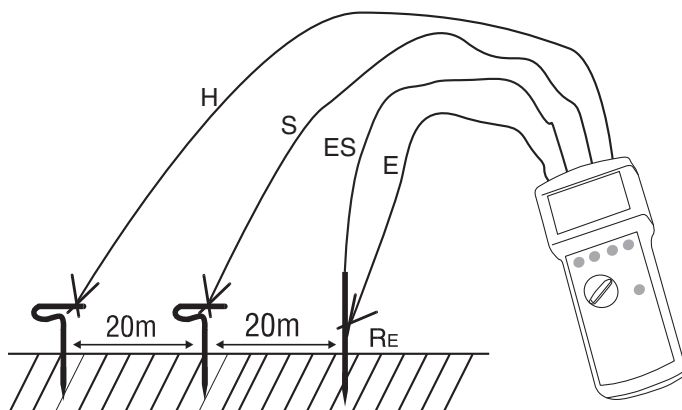
Figura 6: misurazione quadripolare
