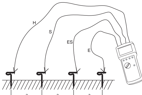
Ilustración 7: Resistencia específica de puesta a tierra
