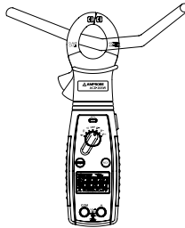
Abb. 3 Messen von Wechselstromstärke 12
