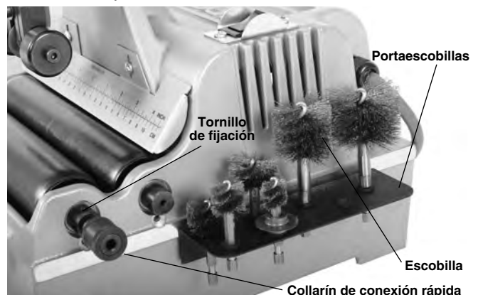
Figura 4 – Collarín
