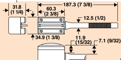
98221 Swivel 88221
