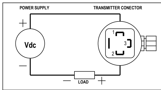
Fig. 02 – Wiring Diagram
