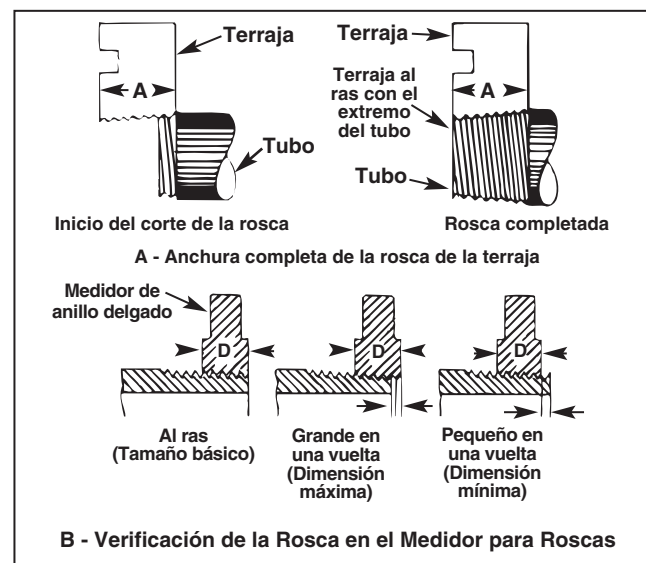
Figura 14 – Verificación de la longitud de la rosca
