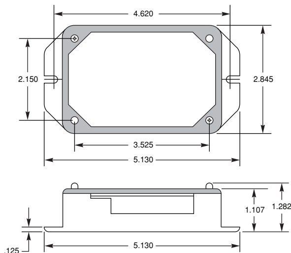
Figura 1 – Dimensiones del Medidor Mini, en pulgadas
