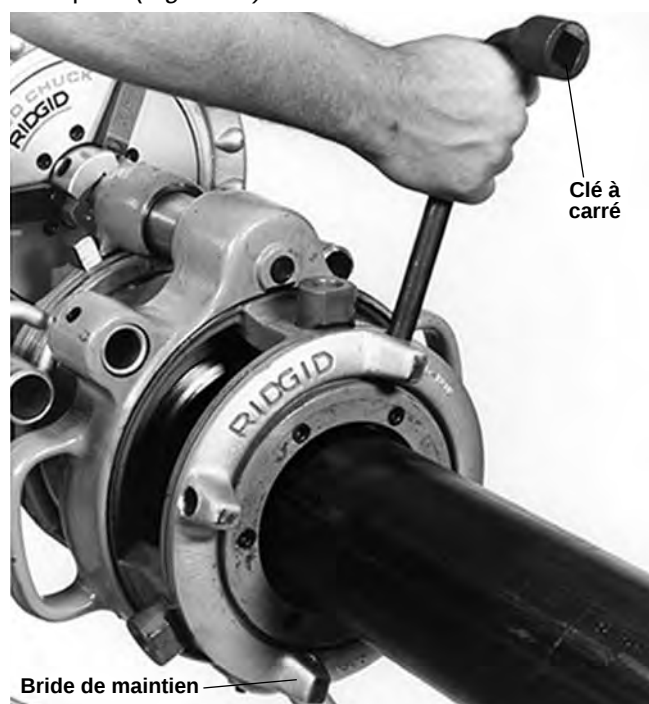
Figure 20 – Serrage de la bride de maintien
