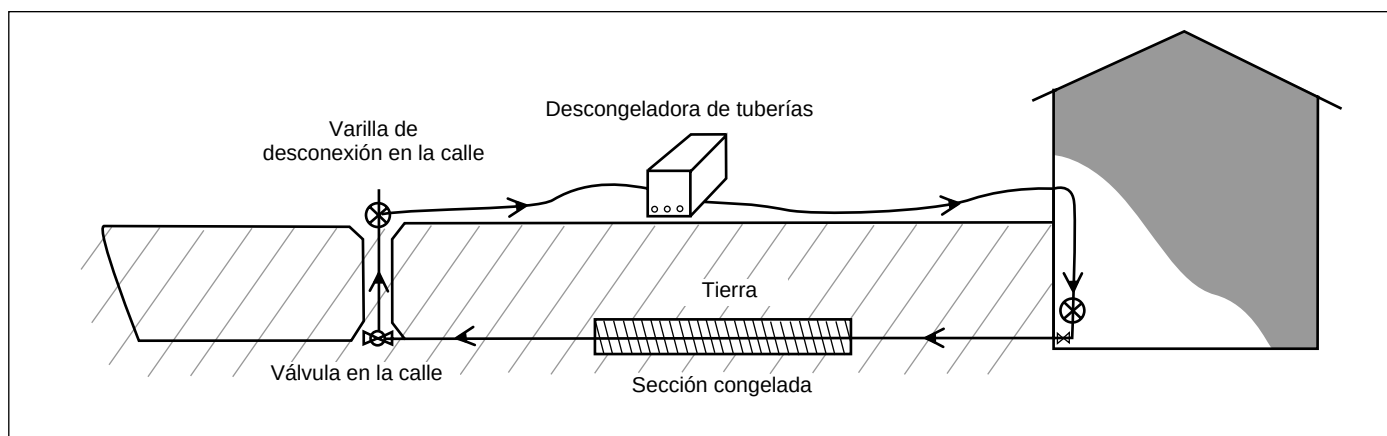
Figura 2 – Descongelación de tuberías principales de servicio público
