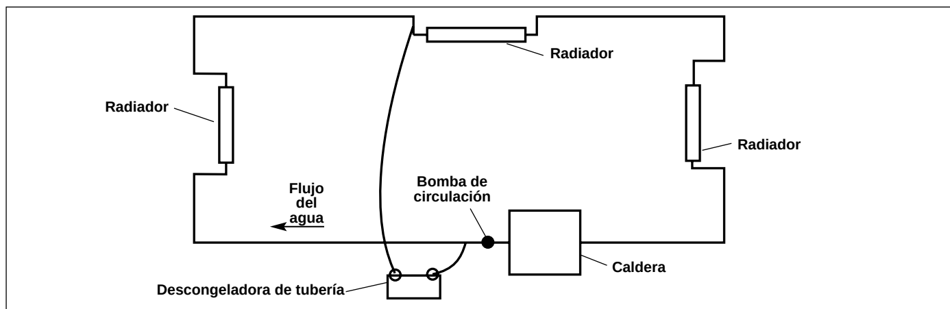
Figura 5 – Red de zona única
