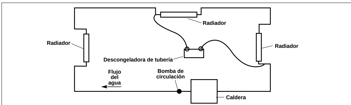
Figura 6 – Red de zona única
