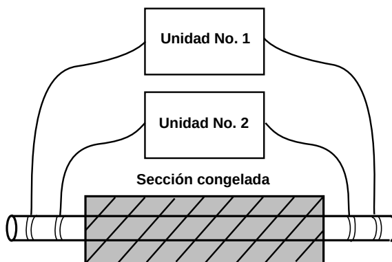
Figura 9 – Instalación en paralelo
