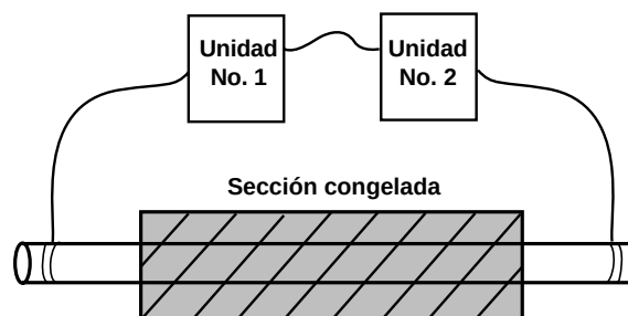
Figura 8 – Instalación en serie
