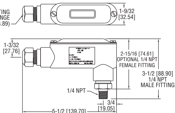
-CH Conduit Housing
