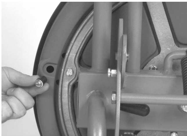
Figura 13 – Tapón de tornillo en agujero para desaguar el tambor
