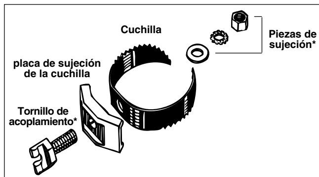
Figura 2 – Ensamblaje de la barrena cortadora
