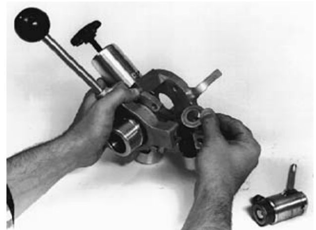
Figura 17 – Introduzca dos arandelas espaciadoras cuando emplee cable de \frac{5}{8} pulg.
