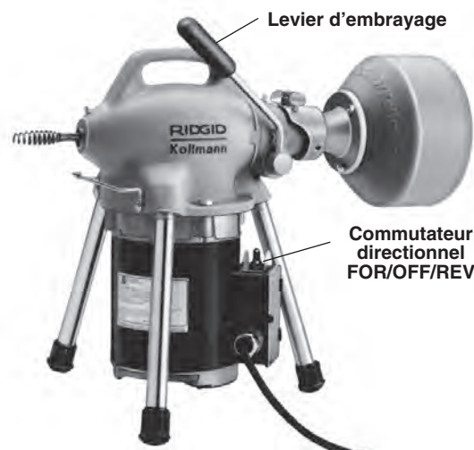
Figure 1 – Dégorgeoir K-50
