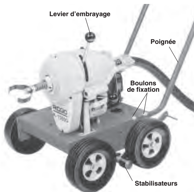
Figure 1 – Dégorgeoir K-1500G
