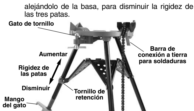
Figura 2 – Ajuste de la tensión de las patas del trípode (460-12)
