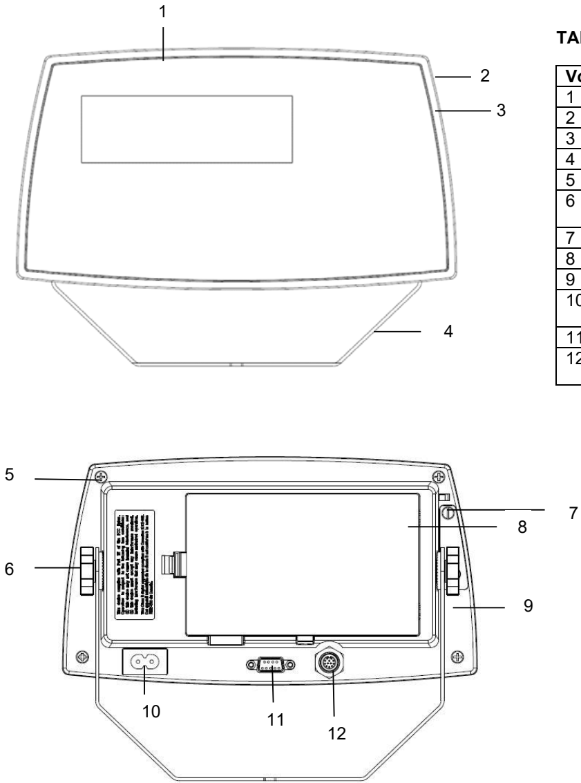
Figura 1-1 Indicatore TD52P
