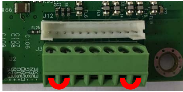
Abbildung 2-4 Jumpverbindungen
