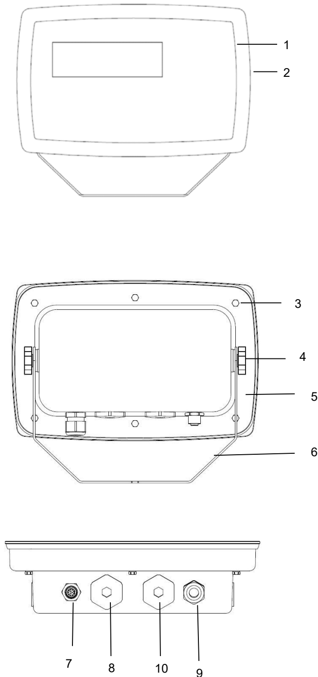
Figure 1-2 Indicateur TD52XW
