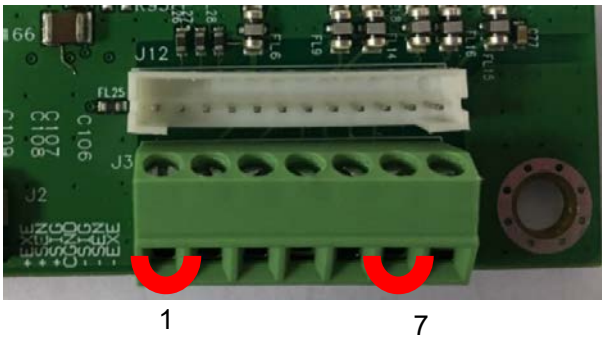
Figura 2-4 Collegamenti Ponticello
