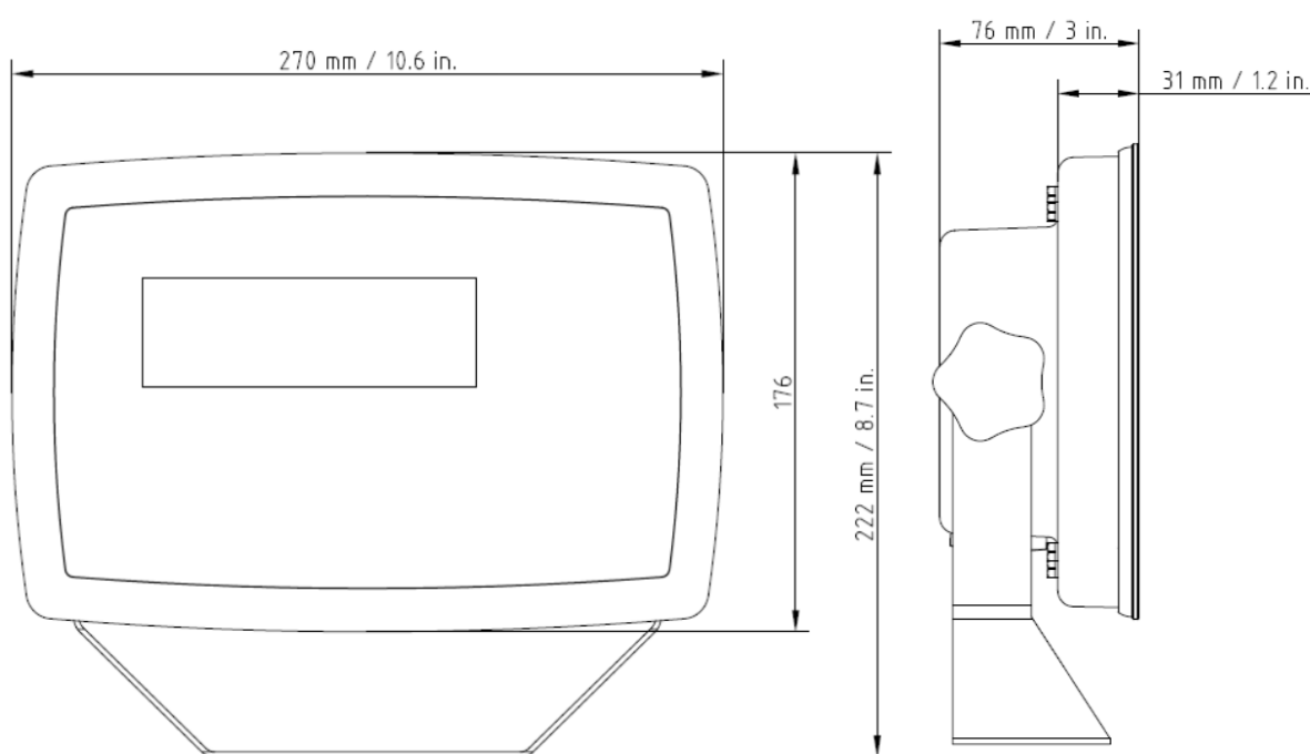
TD52XW
