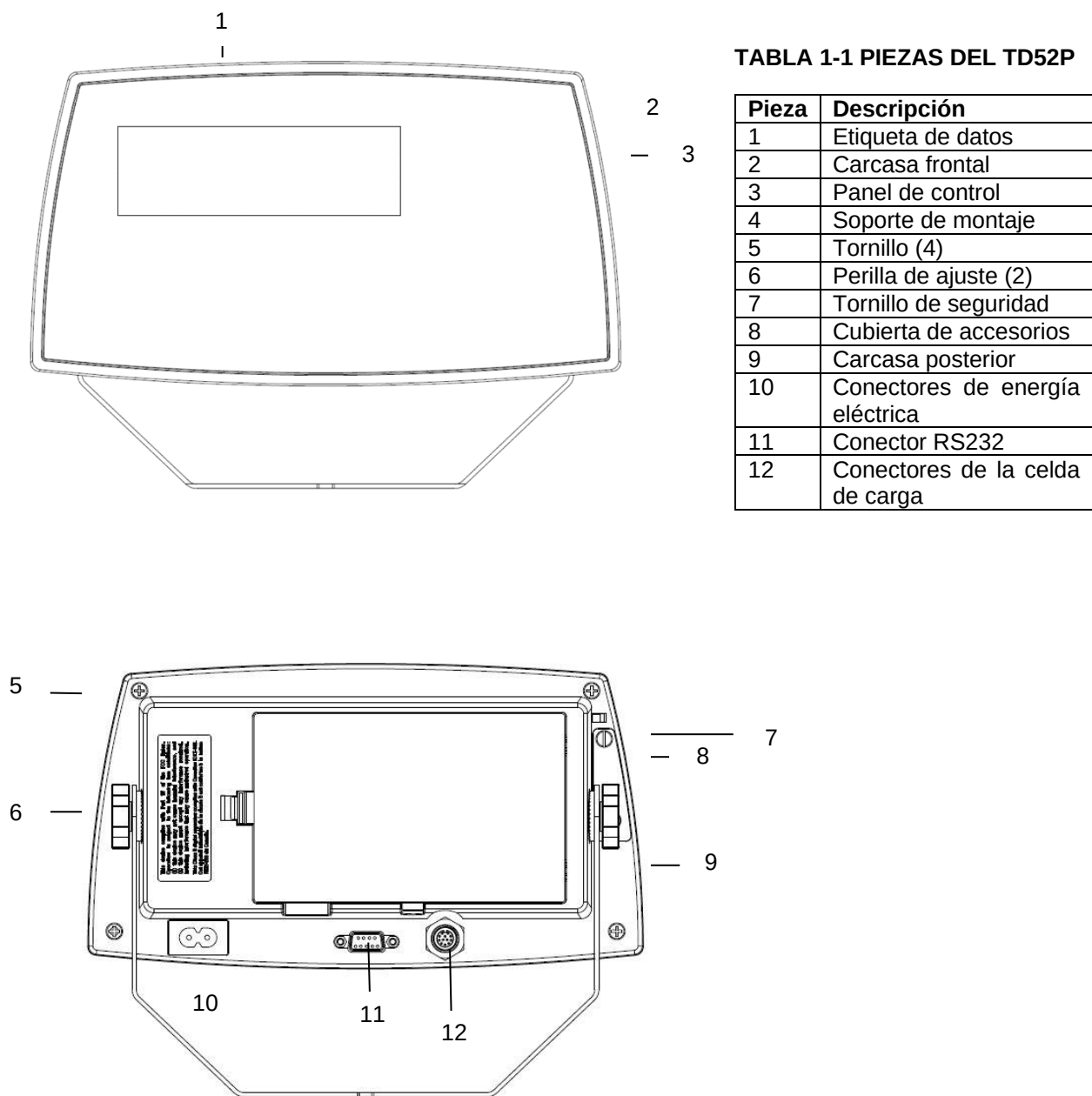
Figura 1-1 Indicador TD52P
