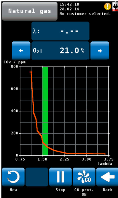
Fig. 53: Tuning Guide
