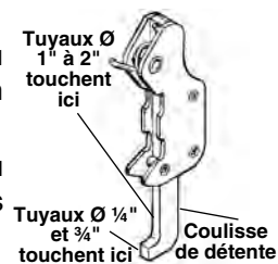
Figure 11 – Réglage de la détente
