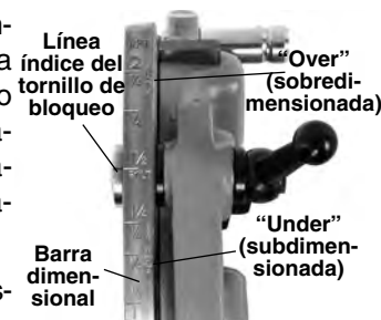
Figura 10 – Ajuste del tamaño de la rosca
