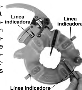
Figura 9 – Inserción de terrajas
