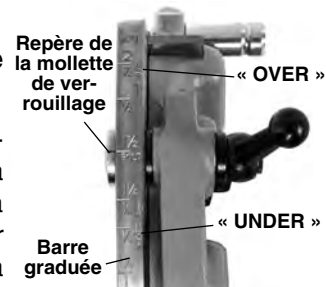
Figure 10 – Réglage du filetage
