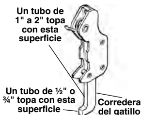
Figura 11 – Posición del gatillo
