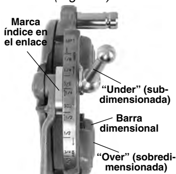
Figura 6 – Ajuste del tamaño de la rosca
