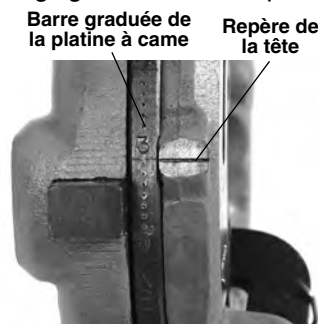
Figure 14 – Réglage du pas de filetage
