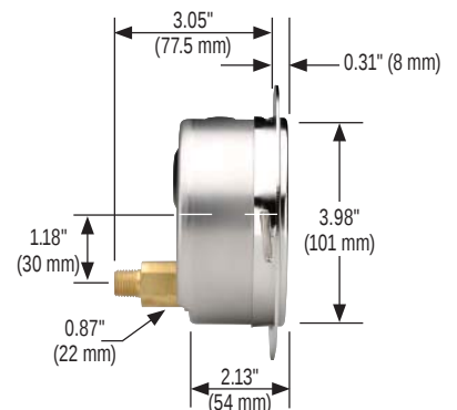
40-911 Front Flange
