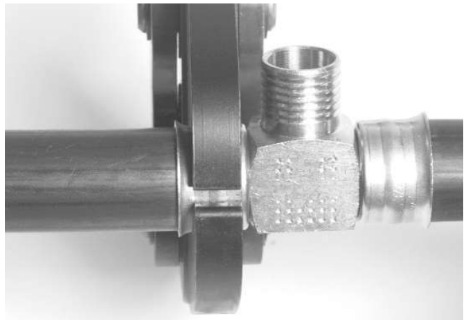
Figura 2 – Mordaza en ángulo recto sobre el acoplamiento PureFlow®
