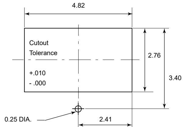
Bezel Panel Cutout
