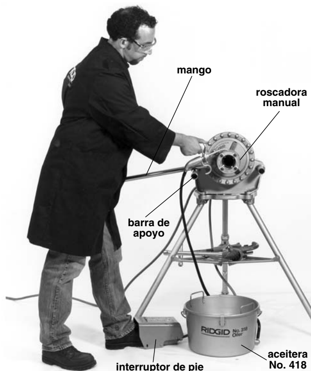
Figura 8 – Roscado con una roscadora manual
