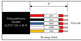
RS-485 Wires
